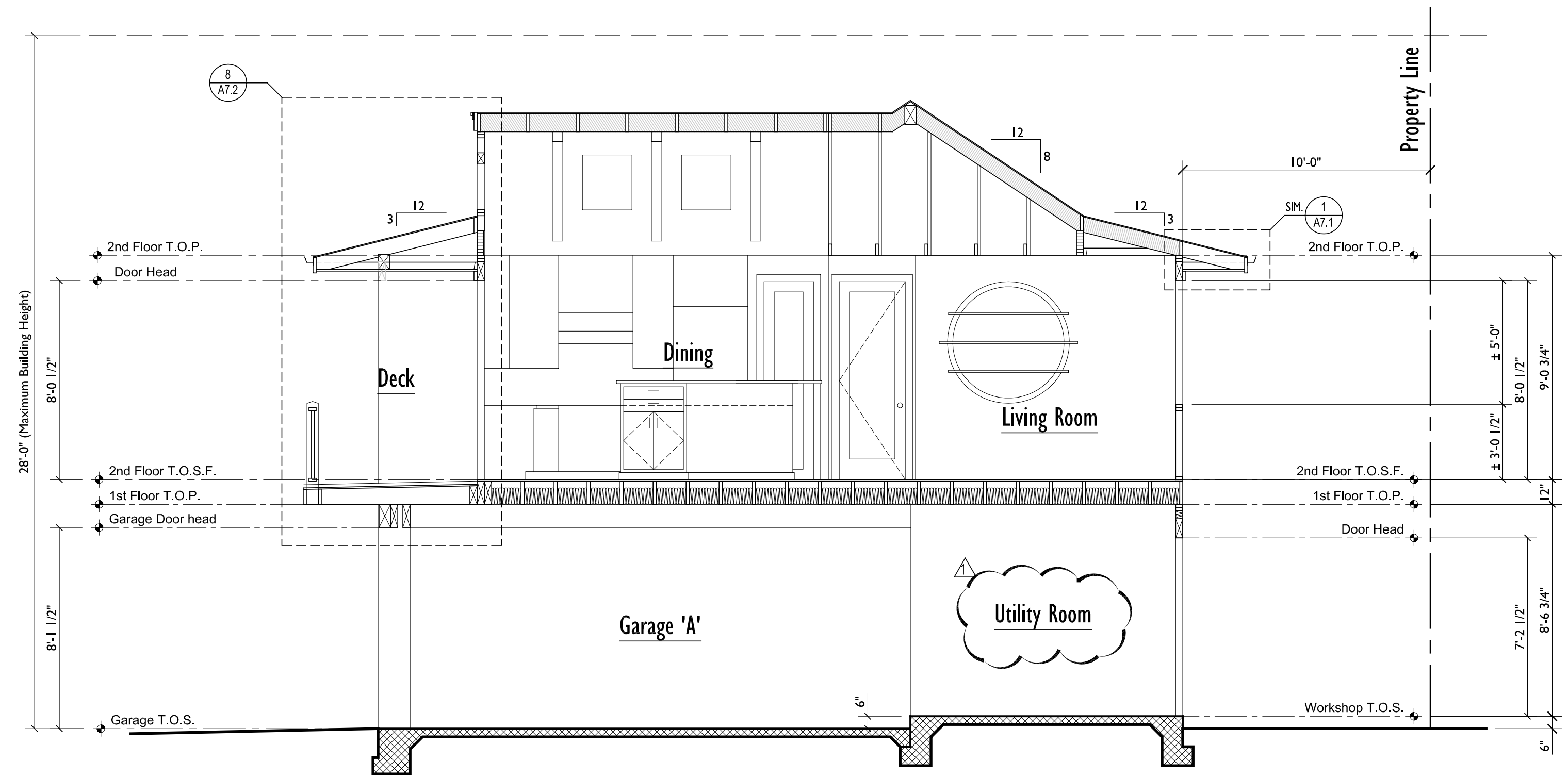
SECTION 'B' SCALE: 1/4" = 1'-0"
