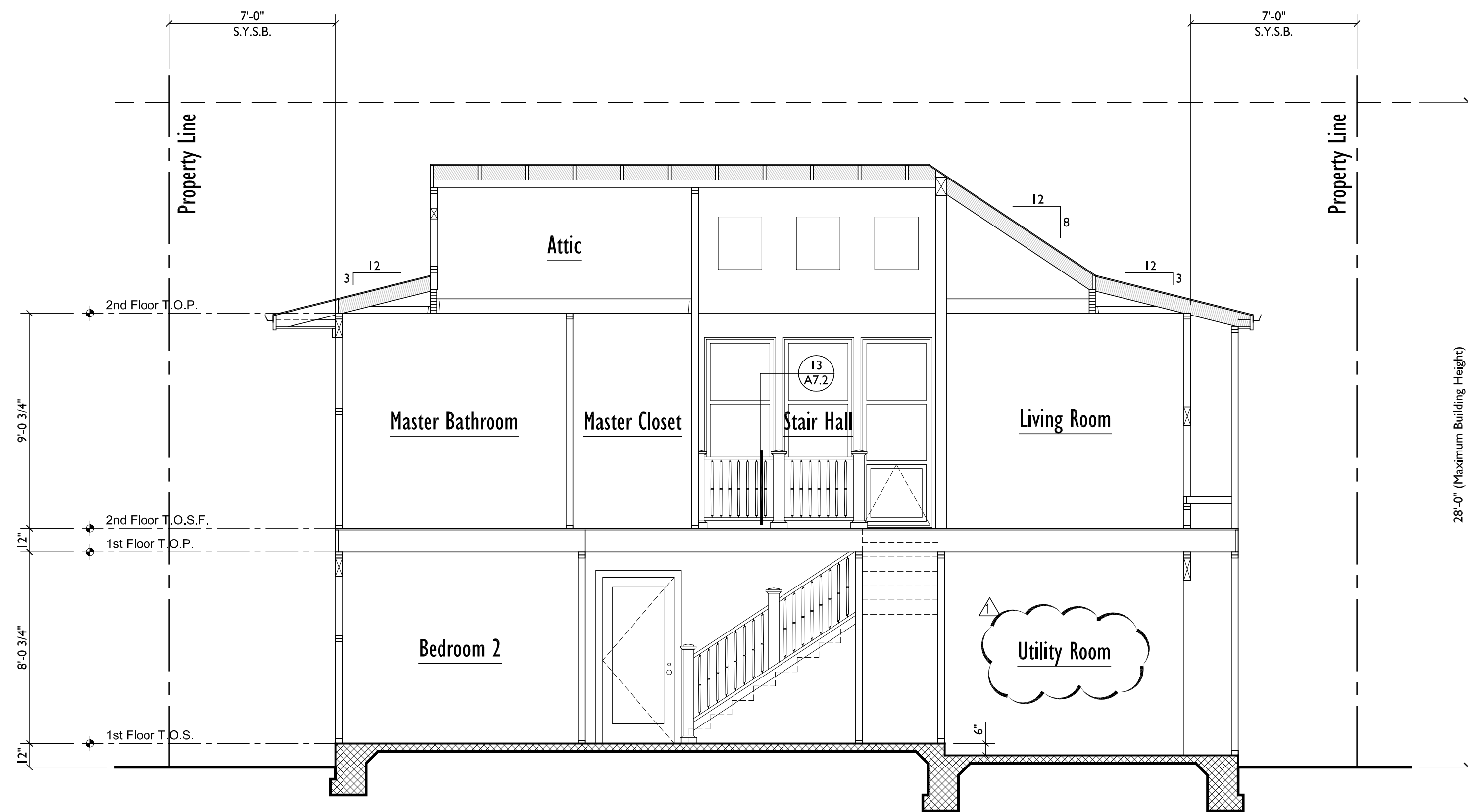
SECTION 'C' SCALE: 1/4" = 1'-0"
