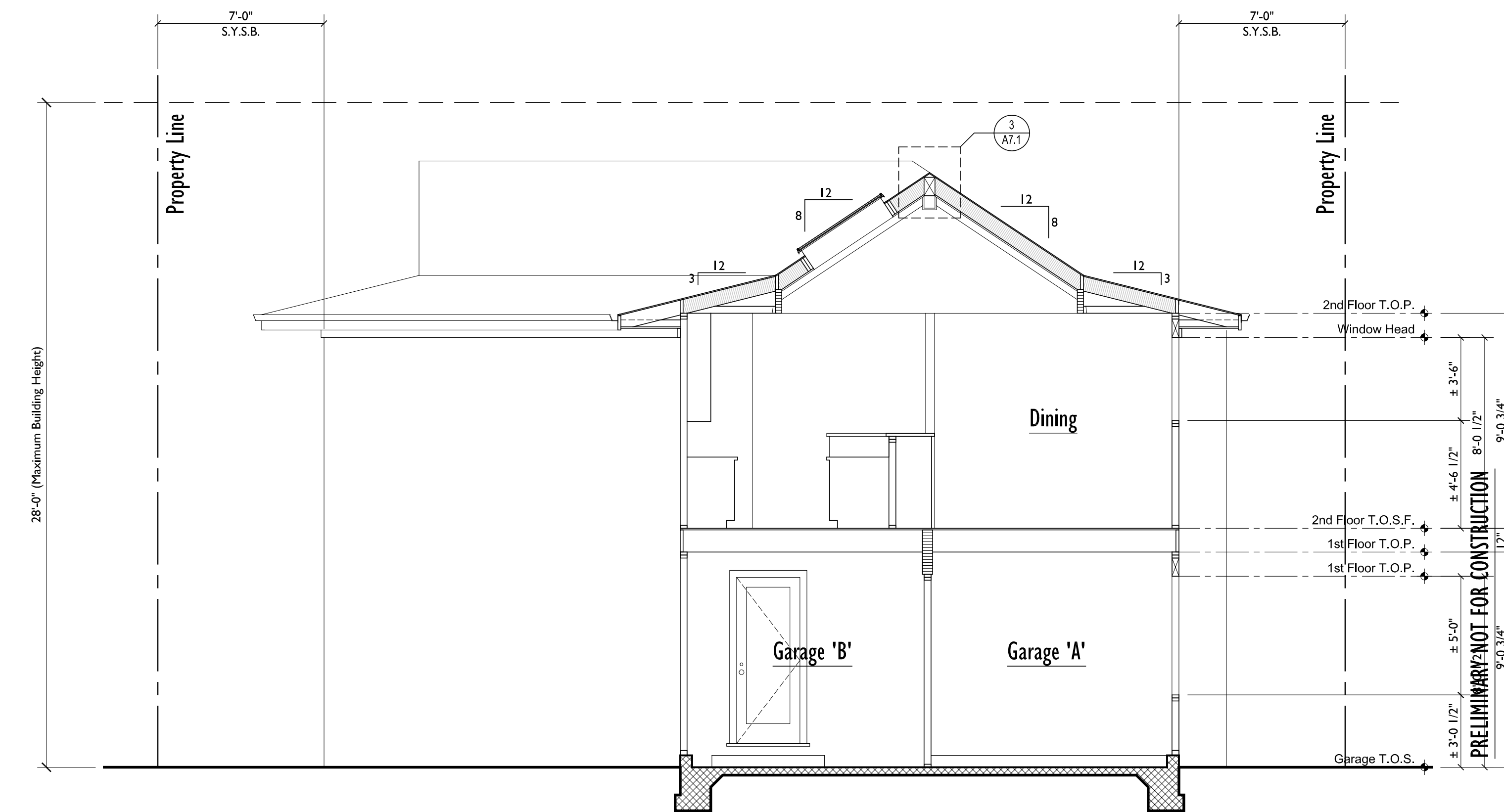
SECTION 'D' SCALE: 1/4" = 1'-0"
